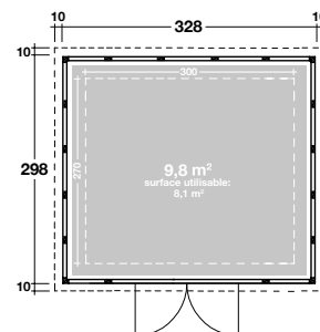
Eleganto 3330 : Dimensions extérieures 328x298 cm - Dimensions intérieures 300x270 cm Hauteur: 219 cm - Pente de toiture: 2°
