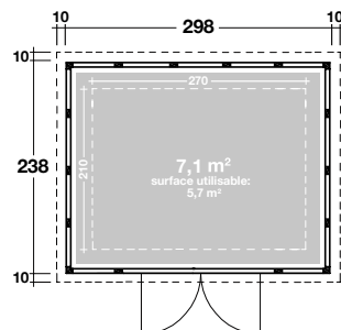
Eleganto 3024 : Dimensions extérieures 298x238 cm - Dimensions intérieures 270x210 cm Hauteur: 219 cm - Pente de toiture: 2°
