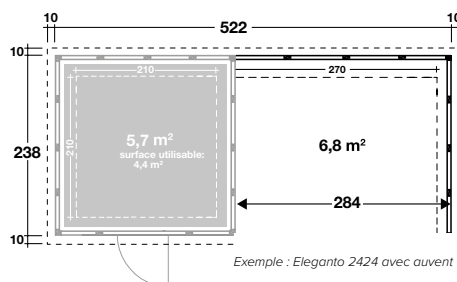
Auvent Lounge Eleganto : Dimensions extérieures 284x238 cm - Dimensions intérieures 270x210 cm. Uniquement combinable avec les modèles ELEGANTO : • 2424 Hauteur: 219 cm • 2724 Pente de toiture: 2° • 3024
