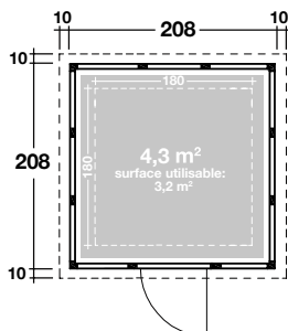
Eleganto 2121 : Dimensions extérieures 208x208 cm - Dimensions intérieures 180x180 cm Hauteur: 219 cm - Pente de toiture: 2°
