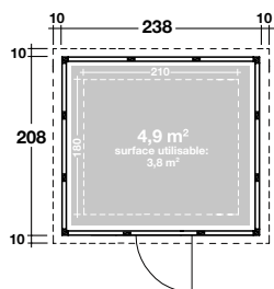
Eleganto 2421 : Dimensions extérieures 238x208 cm - Dimensions intérieures 210x180 cm Hauteur: 219 cm - Pente de toiture: 2°
