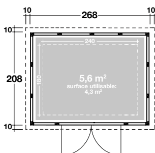
Eleganto 2721 : Dimensions extérieures 268x208 cm - Dimensions intérieures 240x180 cm Hauteur: 219 cm - Pente de toiture: 2°
