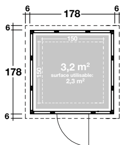
Eleganto 1818 : Dimensions extérieures 178x178 cm - Dimensions intérieures 150x150 cm Hauteur: 207 cm - Pente de toiture: 2°
