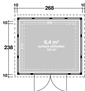
Eleganto 2724 : Dimensions extérieures 268x238 cm - Dimensions intérieures 240x210 cm Hauteur: 219 cm - Pente de toiture: 2°
