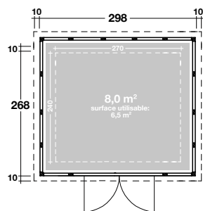
Eleganto 3027 : Dimensions extérieures 298x268 cm - Dimensions intérieures 270x240 cm Hauteur: 219 cm - Pente de toiture: 2°
