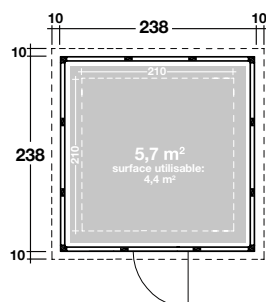
Eleganto 2424 : Dimensions extérieures 238x238 cm - Dimensions intérieures 210x210 cm Hauteur: 219 cm - Pente de toiture: 2°
